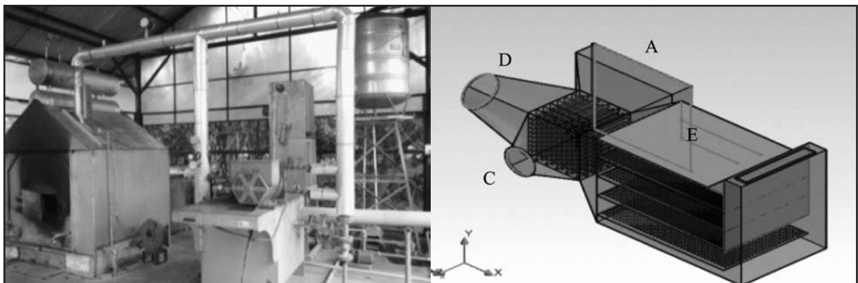
Gambar 2. Model pembangkit listrik tenaga uap (kiri) dan model pengeringan (kanan)
