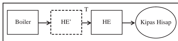
Gambar 6. Skema modifikasi penambahan heat exchanger penurun suhu.
