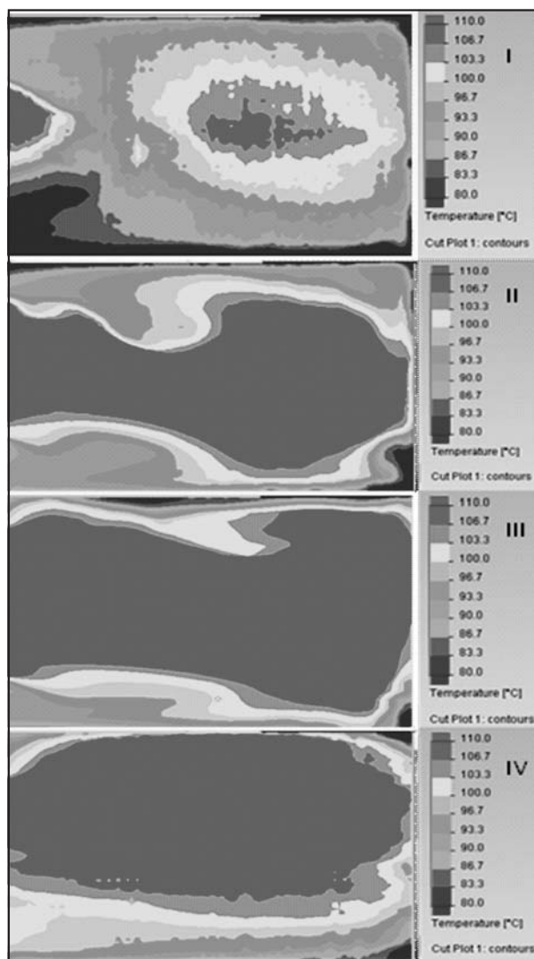
Gambar 10. Kontur suhu pada setiap rak pada frekuensi 25 Hz.
