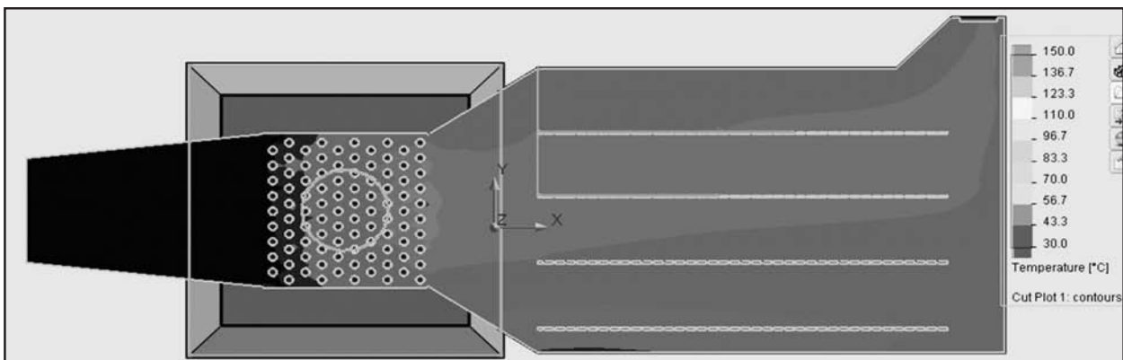
Gambar 3. Sebaran Suhu pada ruang pengering sebelum modifikasi.
