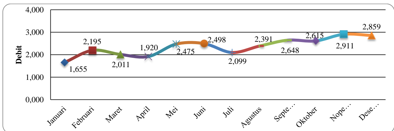
Gambar 1. Grafik debit rata-rata bulanan air sungai Lubuk Paraku tahun 2008 – 2011.
