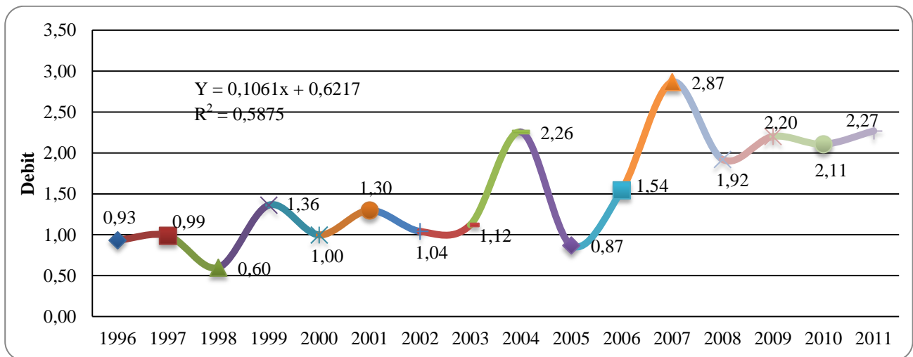
Gambar 2. Grafik rata-rata debit tahunan air sungai Lubuk Paraku tahun 1996-2011.
