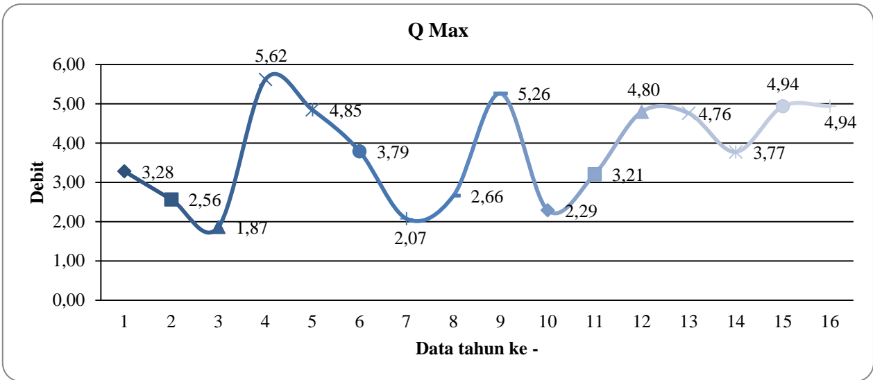
Gambar 3. Grafik debit maksimum sungai Lubuk Paraku dari tahun 1996 – 2011.
